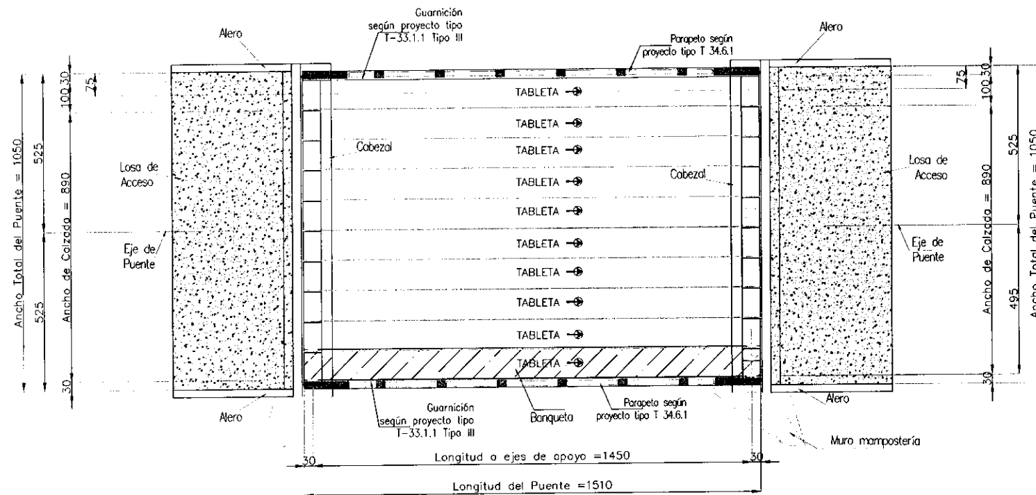
PLANTA DE PUENTE GEOMETRIA esc. 1:100
